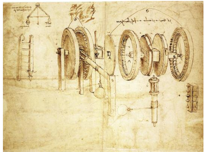
Leonardo da Vinci - Studi sull'igrometro e sulle ruote dentate (1485) Milano, Biblioteca Ambrosiana
